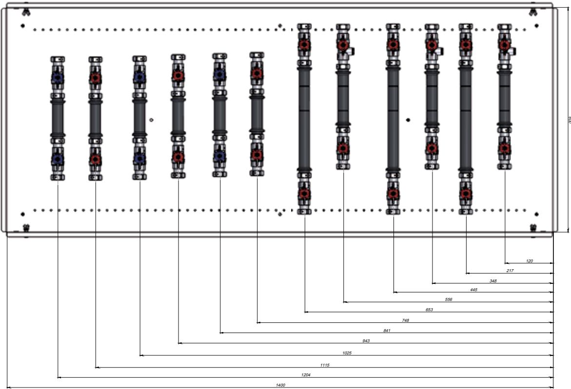
GL2397107 M-BUS 3 USCITE 3 VIE 3/4
