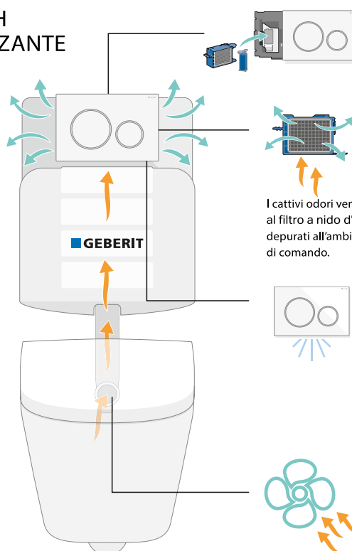
Il nuovo sistema Geberit DuoFresh con la placca di comando Geberit Sigma50.
