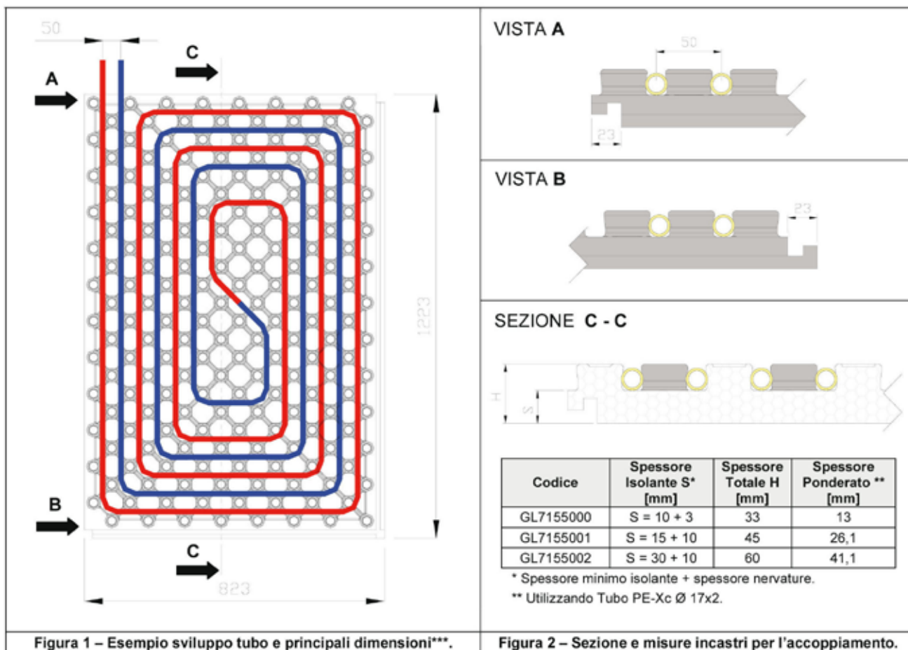
Figura 1 – Esempio sviluppo tubo e principali dimensioni***.
